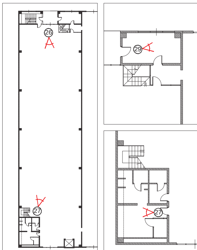
EDIFICIO "A" PIANO TERRA
